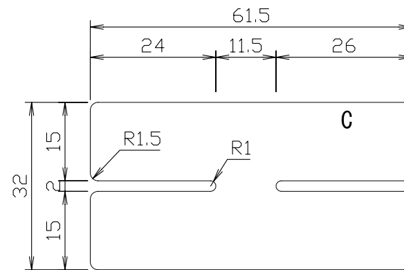
<展開図>
