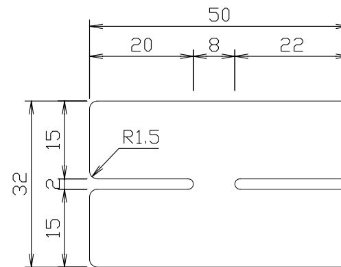
<展開図>
